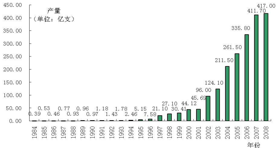
图 1 中国集成电路产量 (1984-2008 年)
